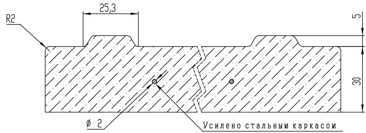
A-A (1:1)
