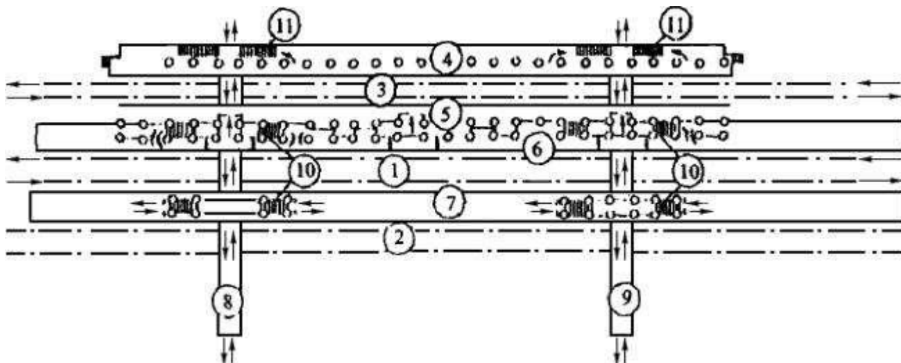
Рисунок В.7 - Организация пересадочного узла при совмещении станций железной дороги и метрополитена с учетом потребностей инвалидов
