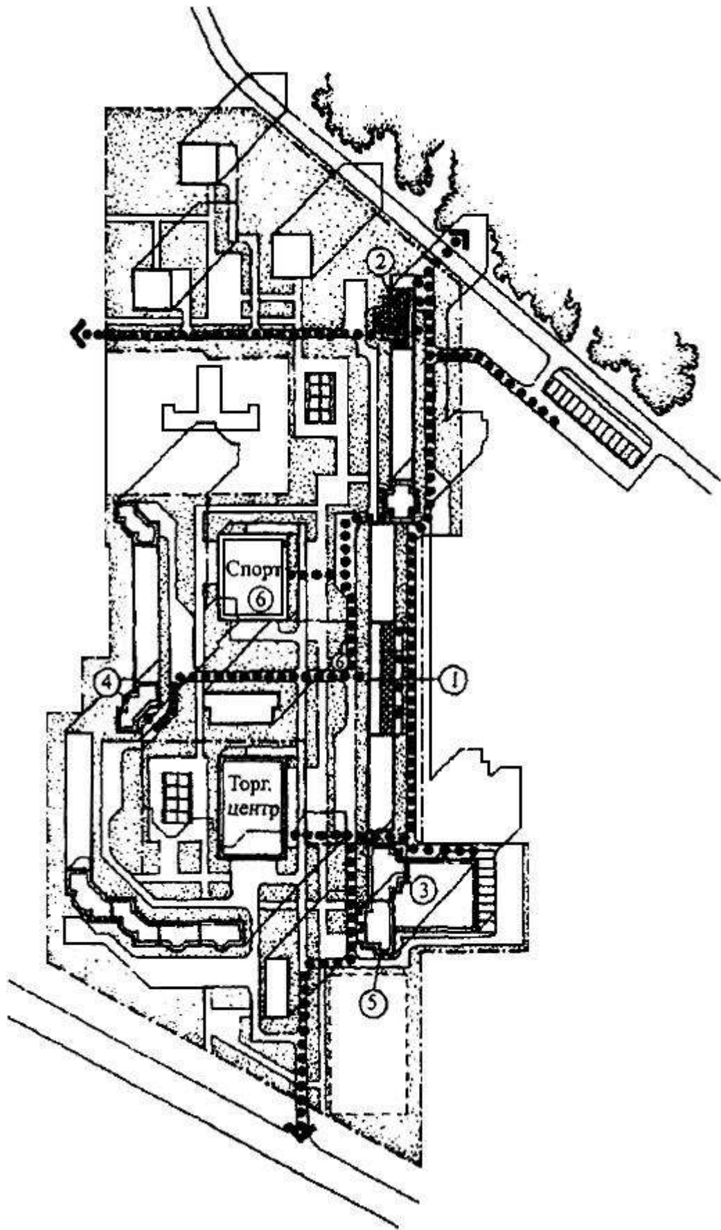
1 - группа квартир с приквартирными участками для инвалидов на креслах-колясках в первом этаже многоквартирного дома после его капитального ремонта и модернизации; 2 - квартиры повышенной комфортности для инвалидов в пристройках, возводимых на
